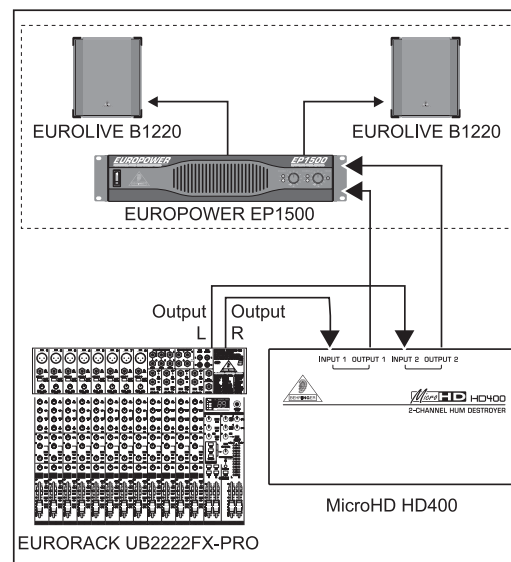
Verkabelung des HD400
